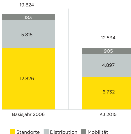
CO 2 -Emissionen in Tonnen
